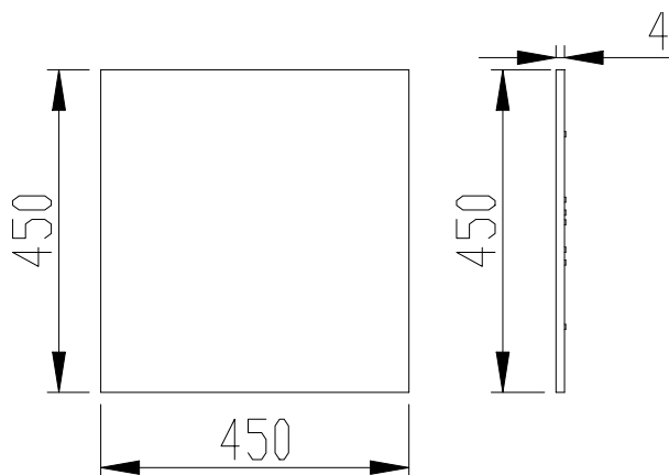
(图4) 铝散热板尺寸图
